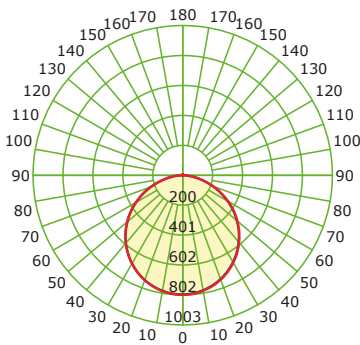
CURVA FOTOMETRICA
